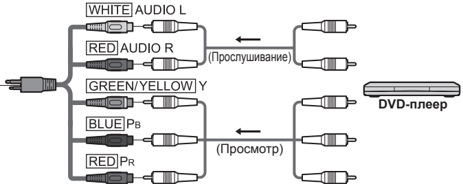
Адаптер AV2 (COMPONENT / VIDEO) (входит в комплект поставки)
