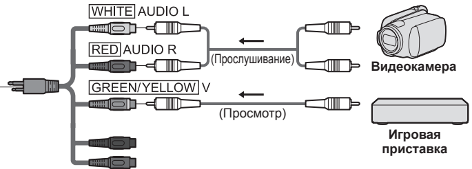
Адаптер AV2 (COMPONENT / VIDEO) (входит в комплект поставки)
