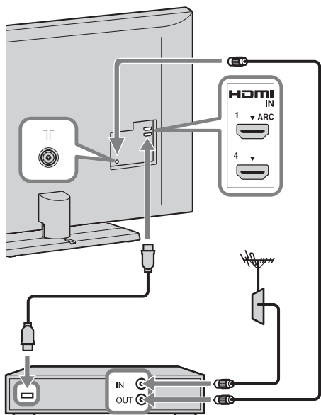
Телеприставка/записывающее устройство (например, DVD-рекордер)
