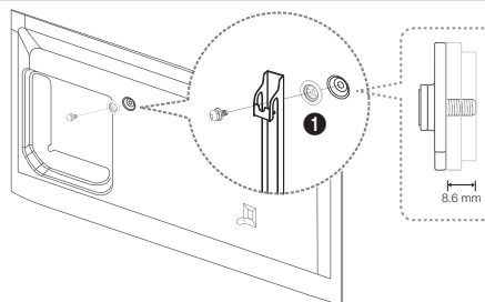
Вариант Б. Установка настенных креплений других производителей
