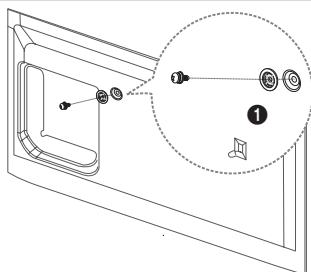
Вариант А. Установка настенного крепления SAMSUNG
