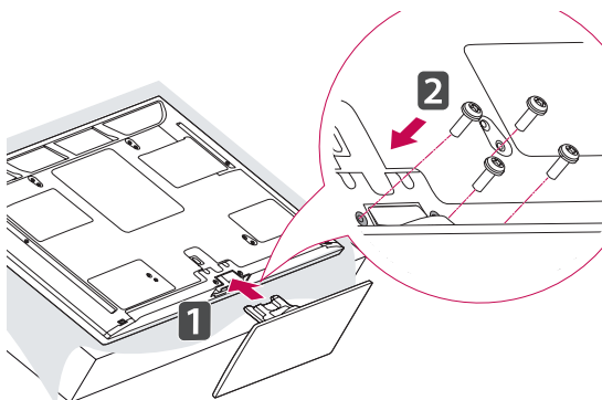
Основание подставки
