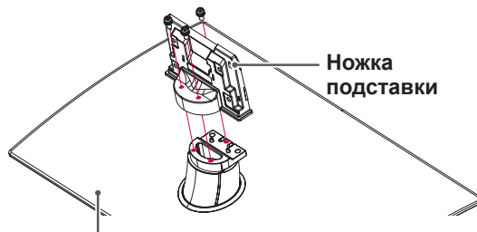
Основание подставки
